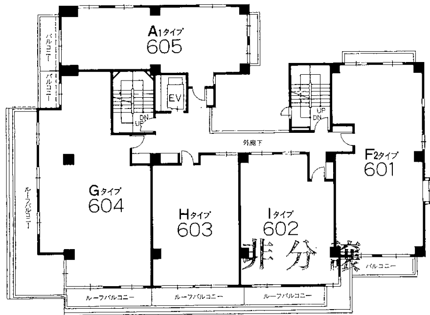
6階平面図
