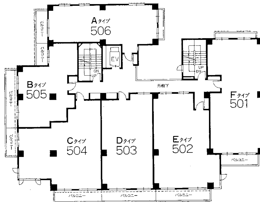
5階平面図
