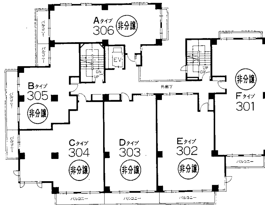
3階平面図
