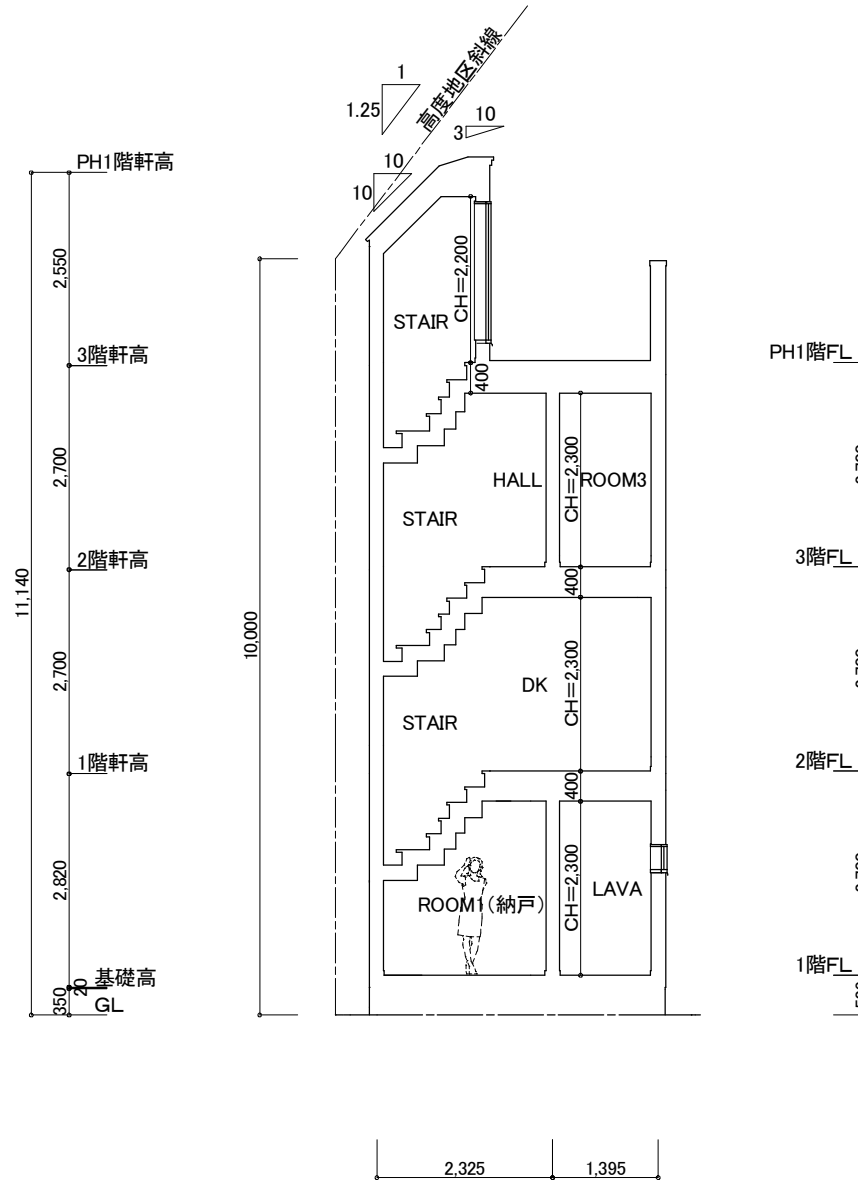
Y - Y' 断面図 S:1/100
