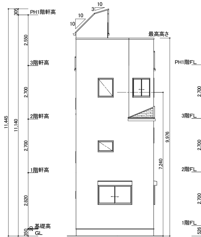
西側 立面図 S:1/100
