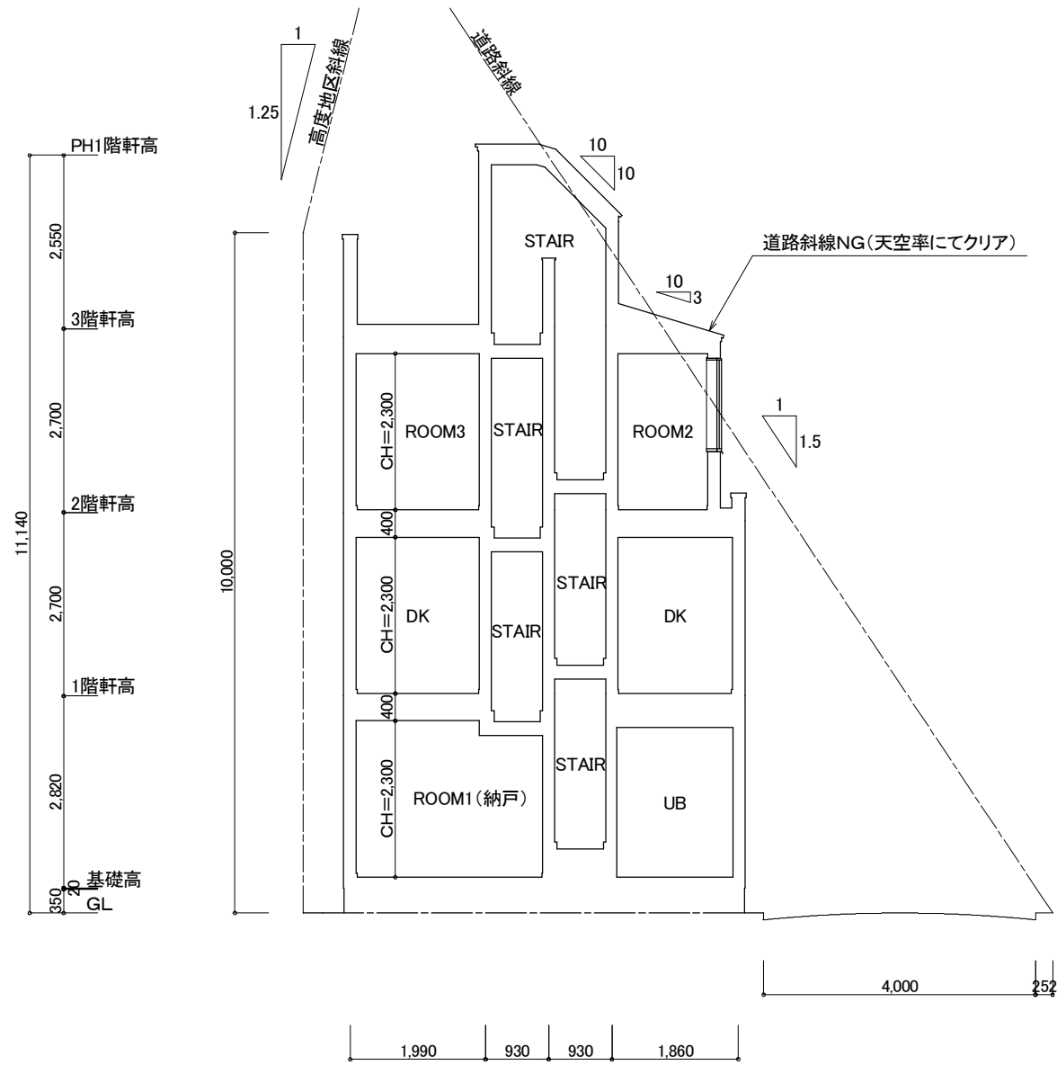
X - X' 断面図 S:1/100
