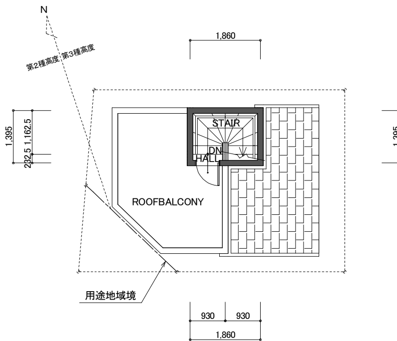
PH1階 平面図 S:1/100
