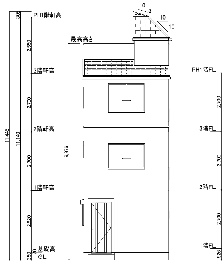
東側 立面図 S:1/100
